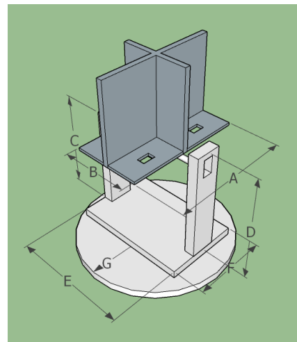
Gambar 2 Desain perangkat hardware
