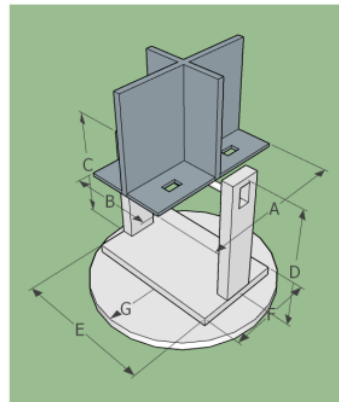
Gambar 2 Desain perangkat hardware
