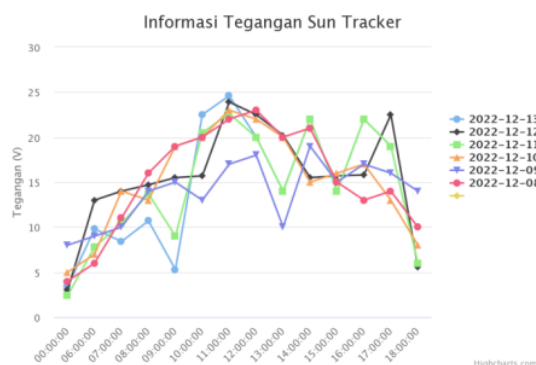
Gambar 18 Grafik tegangan selama 1 minggu
