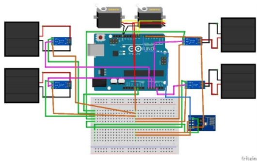
Gambar 5 Rancangan sistem keseluruhan
