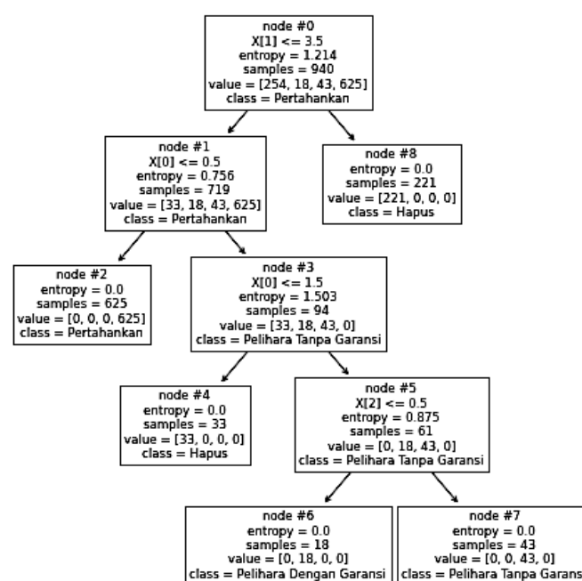
Gambar 5: Pohon keputusan berbasis C5.0
