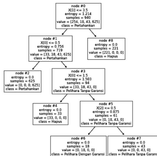
Gambar 5: Pohon keputusan berbasis C5.0
